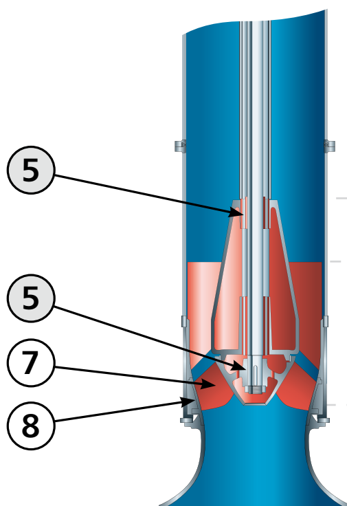
Модульная конструкция извлекаемого типа
